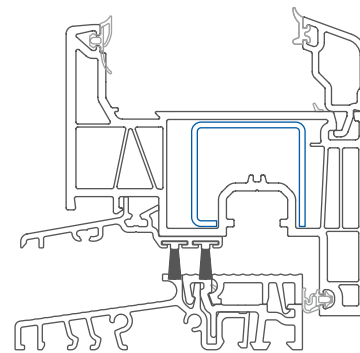
Elegant balkonska vrata z zaobljeno steklitveno letvico Merilo: 1:2
